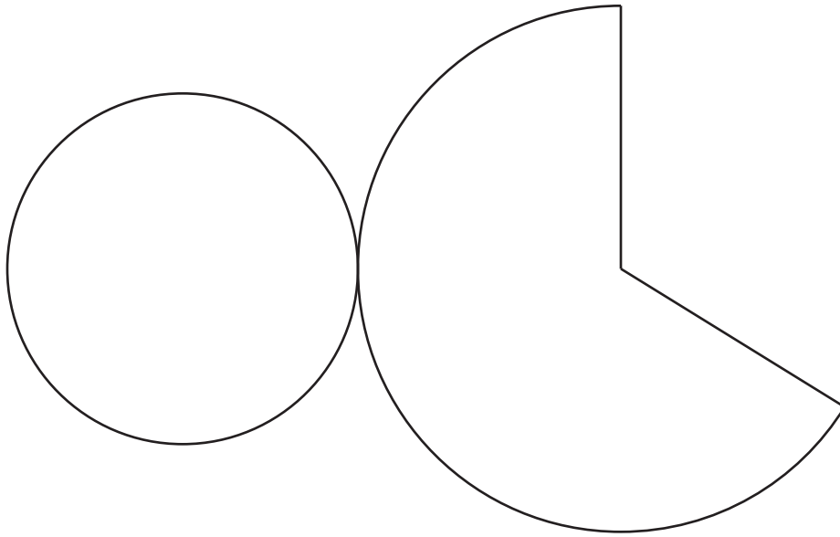
Cone
